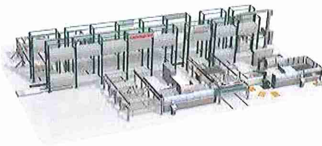
1. FMS-anlæg hos Danpres
